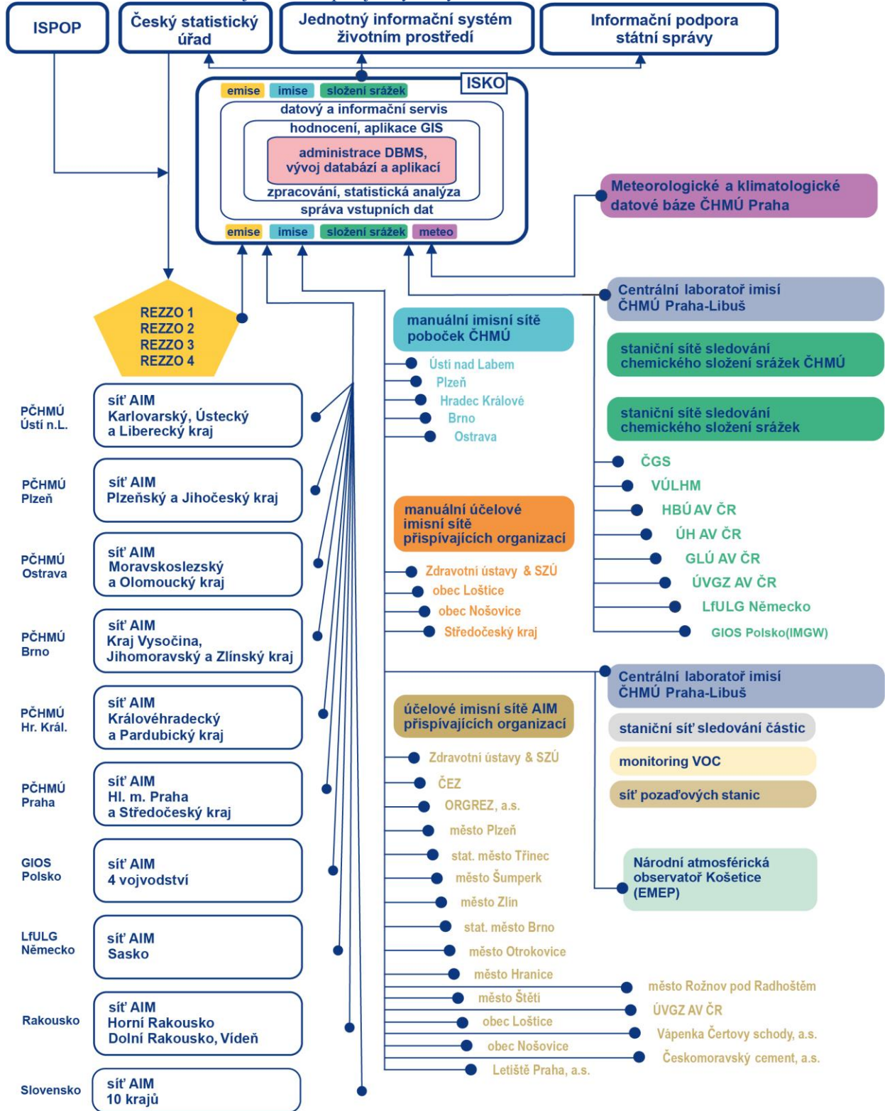
Obr. 1 Schéma vazeb ISKO na zdroje dat a kooperující systémy v roce 2021
