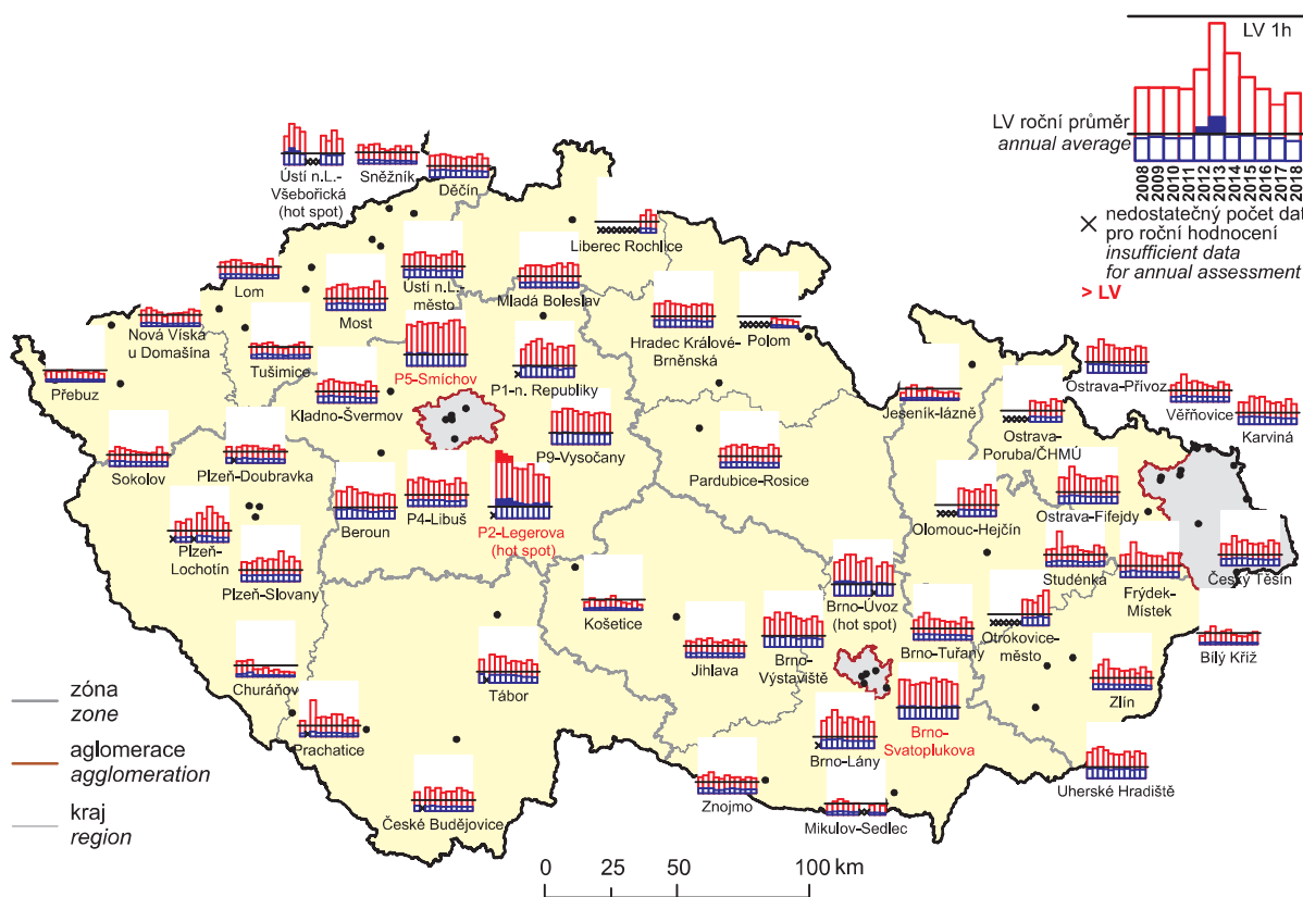
Obr. IV.3.5 19. nejvyšší hodinové koncentrace a roční průměrné koncentrace NO 2 na vybraných stanicích, 2008–2018 Fig. IV.3.5 19 th highest hourly concentrations and annual average concentrations of NO 2 at selected stations, 2008–2018
