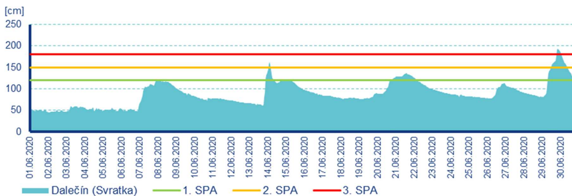
Obrázek 4.7.1 - Hodinové stavy ve vybraných profilech na tocích v povodí Dyje
